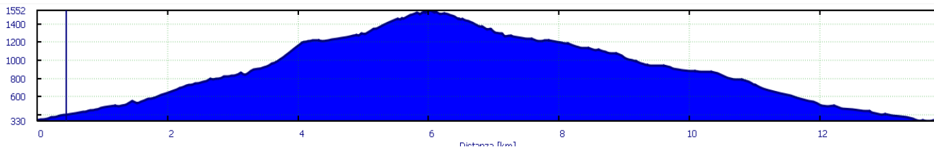
Profilo altimetrico del percorso di escursione
