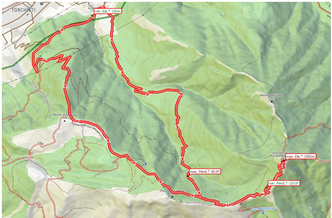
Itinerario di escursione evidenziato in rosso (mappa FreemapSK)
